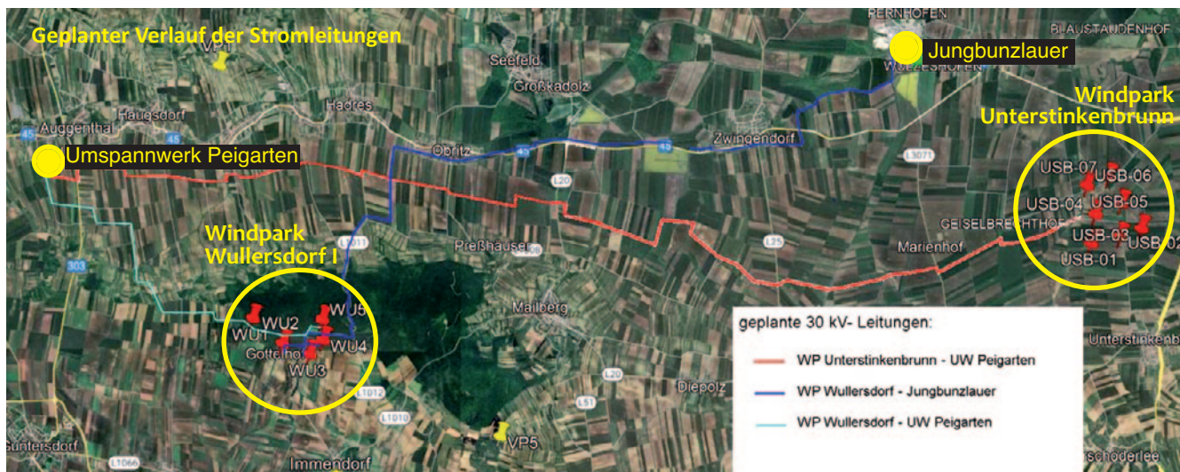
Geplanter Verlauf der Stromableitungen aus den Windparks Wullersdorf I und Unterstinkenbrunn: Irrsinn mit Ansage!
